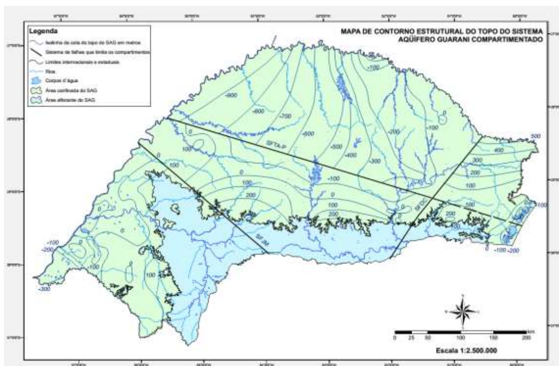
Figura 25. Contorno estrutural do topo do sistema Aquífero Guarani Compartimentado (Machado, 2005).
